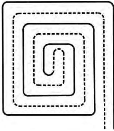
Abbildung 9: Verlegeart Schnecke (nach RAUGEO 2007)
