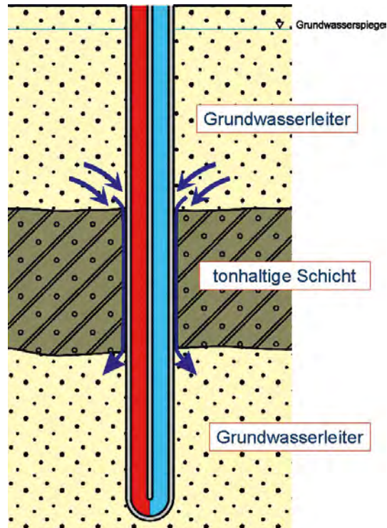
Abbildung 13: Mögliche Wasserwegsamkeiten bei nicht ordnungsgemäß abgedichteter Sonde
