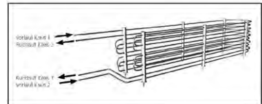
Abbildung 6: U-förmiger, senkrecht verlegter Grabenkollektor (Quelle: Fa. Roth, 2009) – Länge 5 m, Höhe 1 m und Breite 0,8 m
