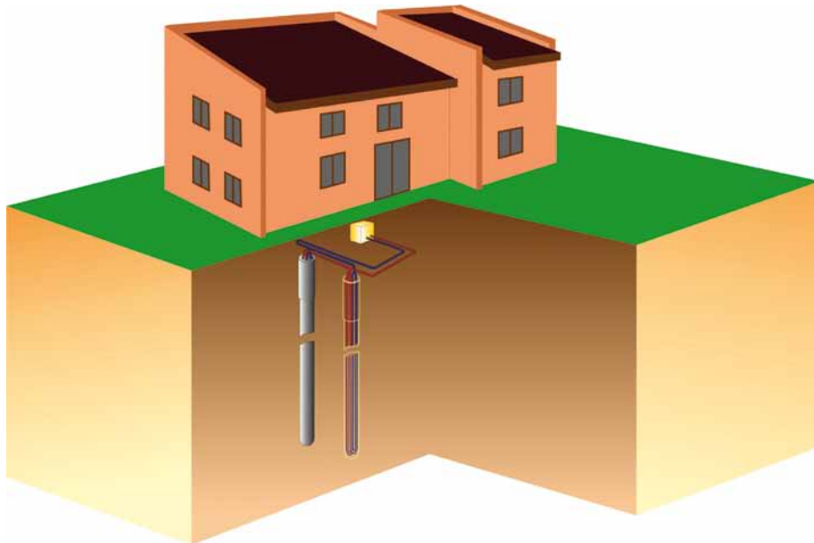
Abbildung 7: Erdwärmesonden
