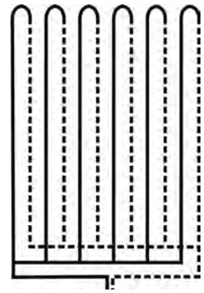
Verlegeart Tichelmann
